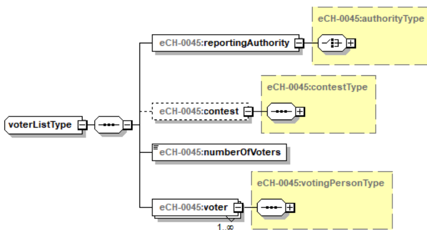
Figure 14: voterList – Liste des électeurs inscrits
