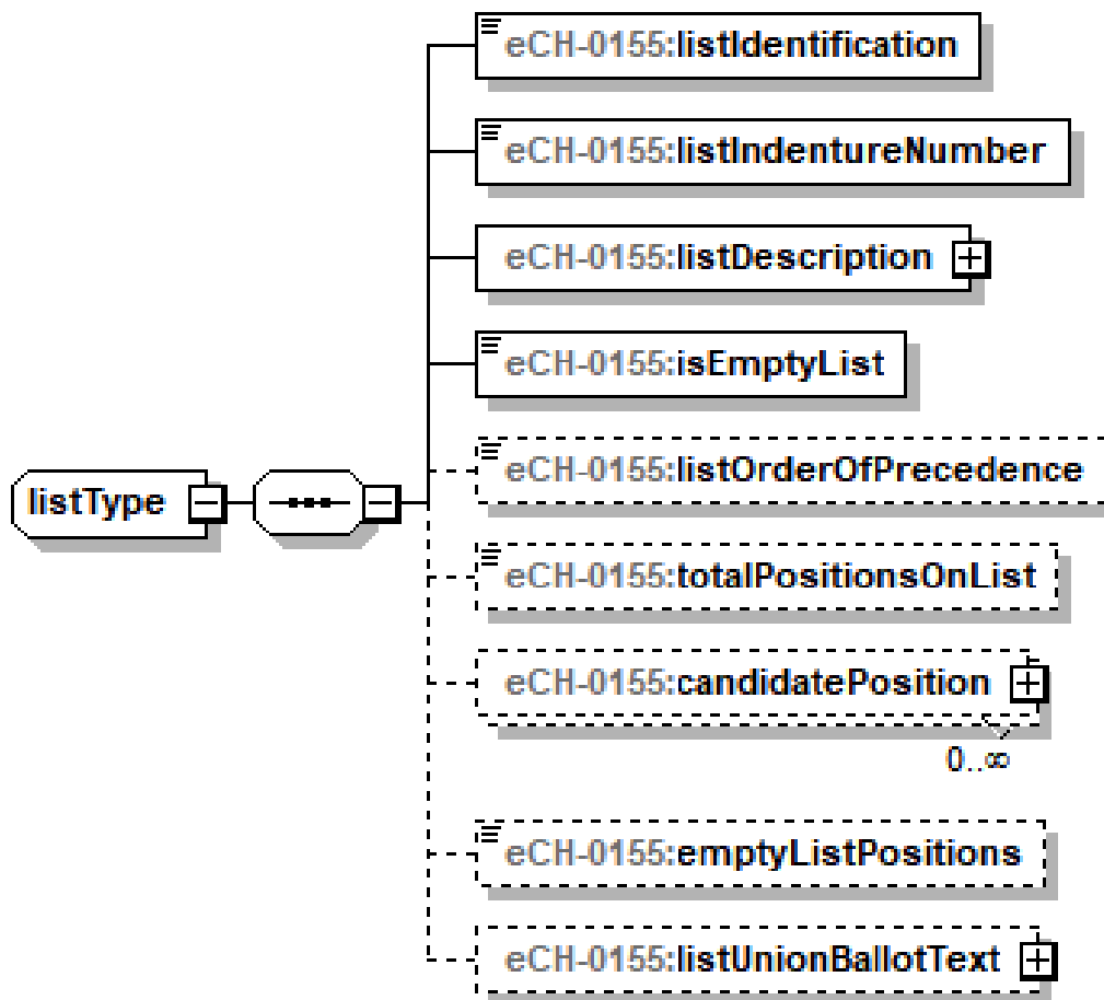
Abbildung 22: Wahlliste – list
