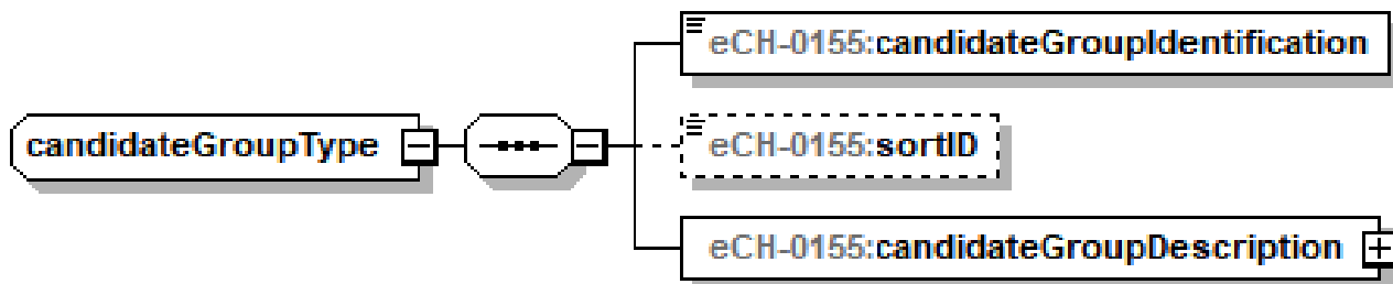
Abbildung 15: Kandidatengruppe – candidateGroup
