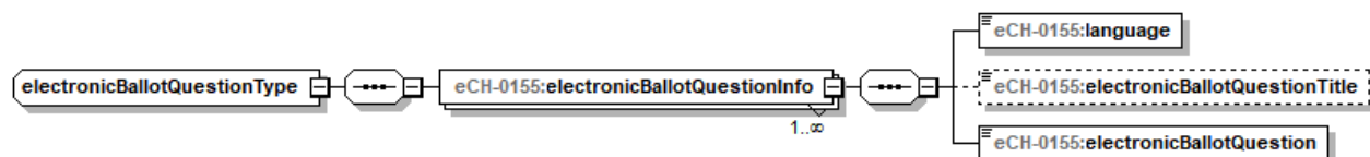
Abbildung 38: Abstimmungsfrage – ballotQuestion
