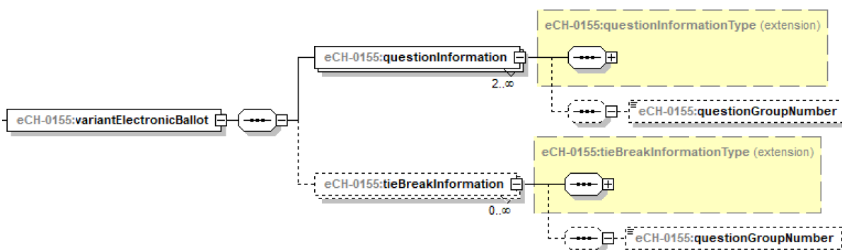
Abbildung 35: Variantenvorlage – variantElectronicBallot
