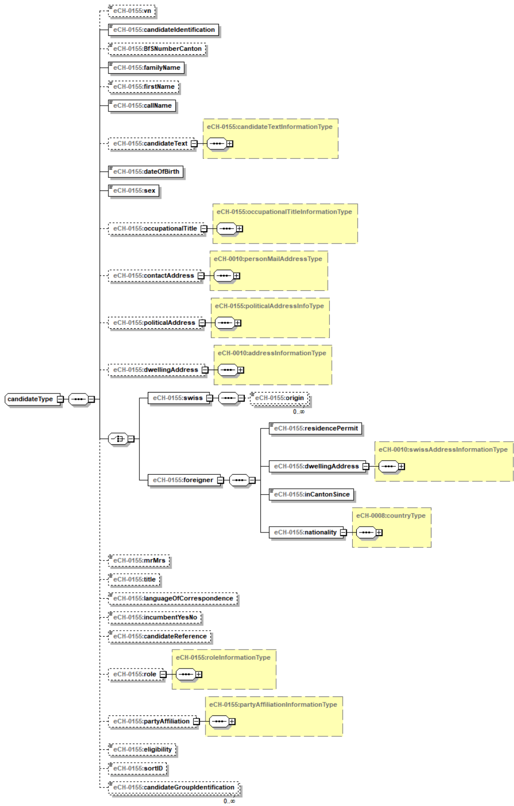
Abbildung 9: Kandidat – candidate
