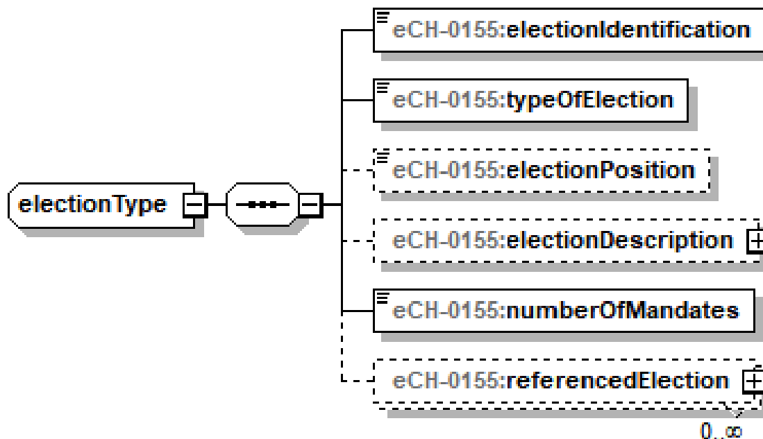
Abbildung 18: Wahl – electionType
