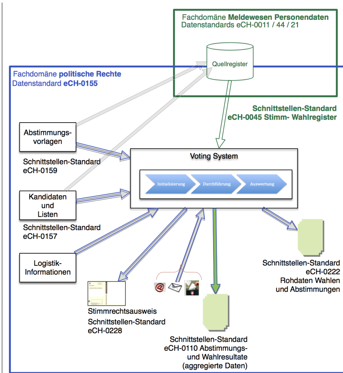
Abbildung 1: Übersicht
