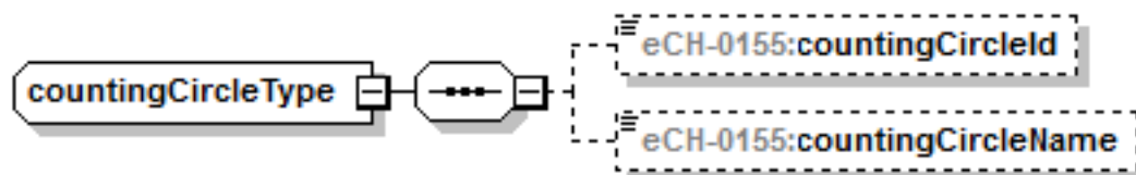
Abbildung 6: Auszählkreis – countingCircle
