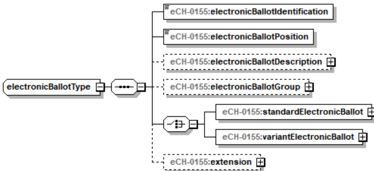
Abbildung 32: Vorlage – electronicBallot
