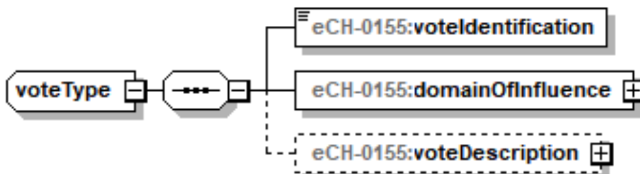
Abbildung 30: Abstimmung – vote
