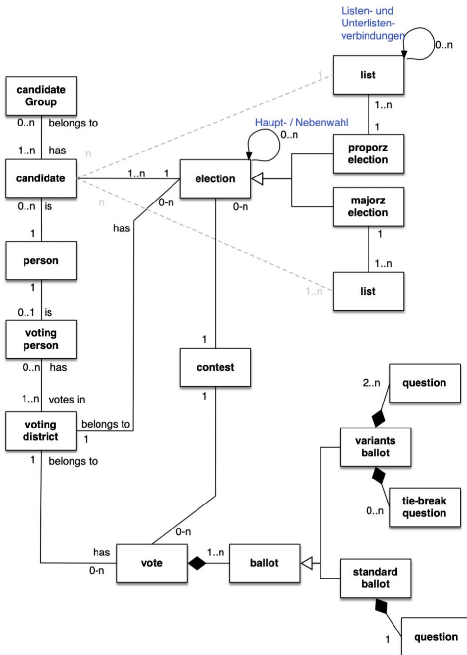
Abbildung 2: Datenmodell
