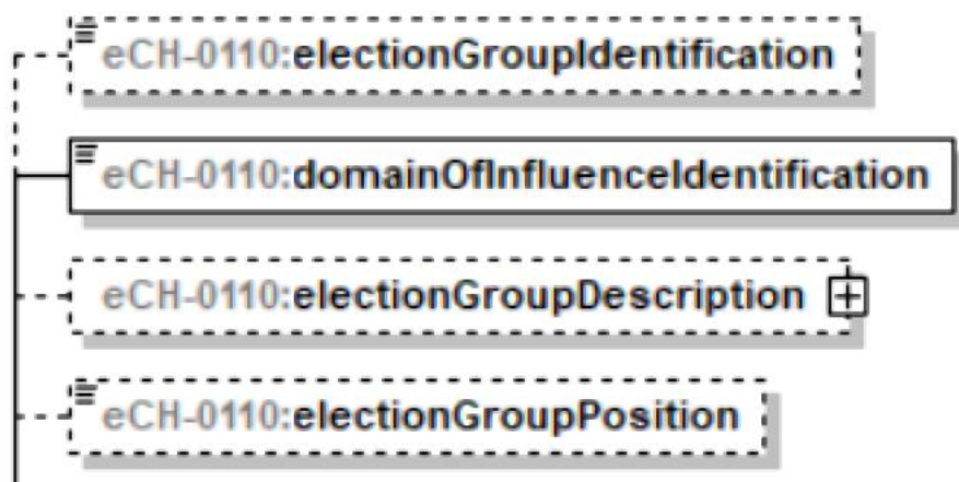
Abbildung 17: Wahlgruppe – electionGroup
