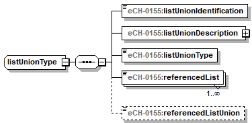
Abbildung 26: Listenverbindung – listUnion
