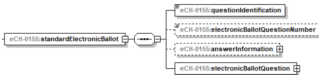
Abbildung 34: Standardvorlage – standardElectronicBallot
