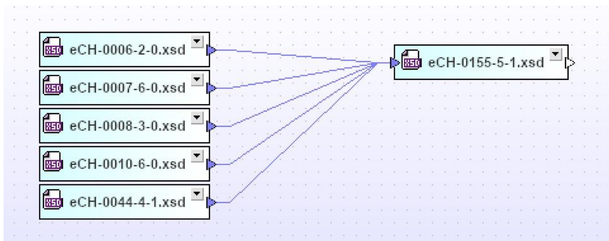
Abbildung 43: Abhängigkeiten
