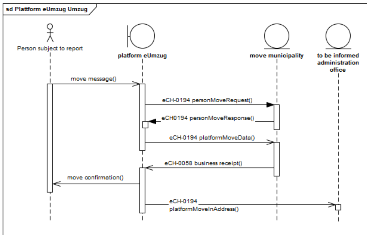
Figure 4: Déménagement
