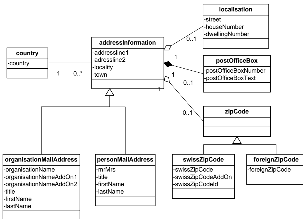
Abbildung 1: UML-Diagramm zur Postadresse
