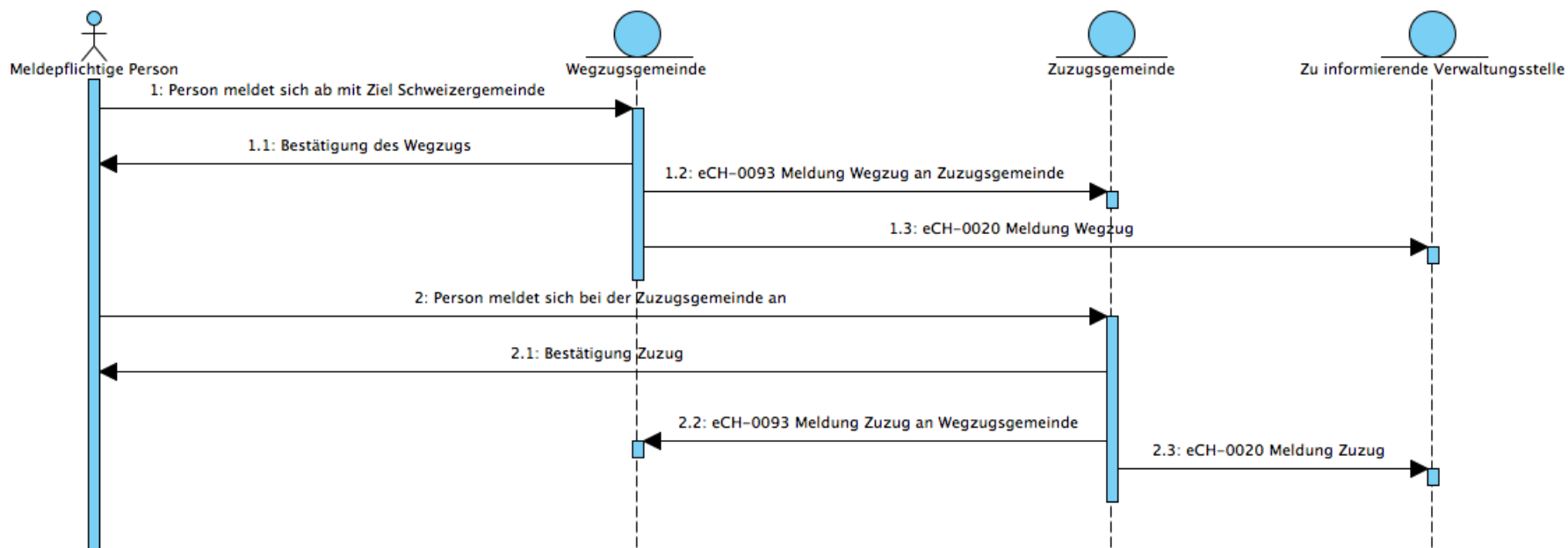
Figure 3: Diagramme UML concernant le processus de départ / arrivée
