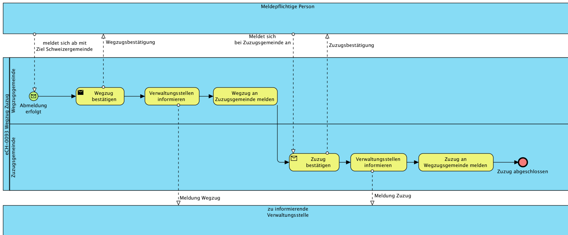
Figure 4: Diagramme BPMN concernant le processus départ / arrivée
