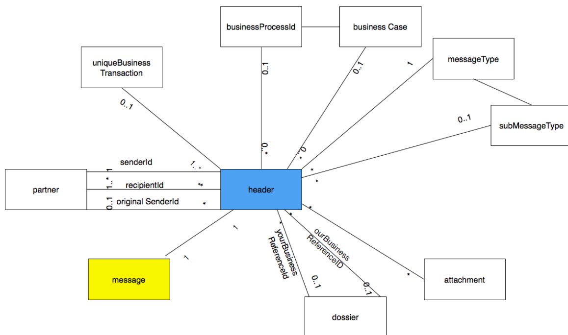
Abbildung 6: Datenmodell eCH-0058
