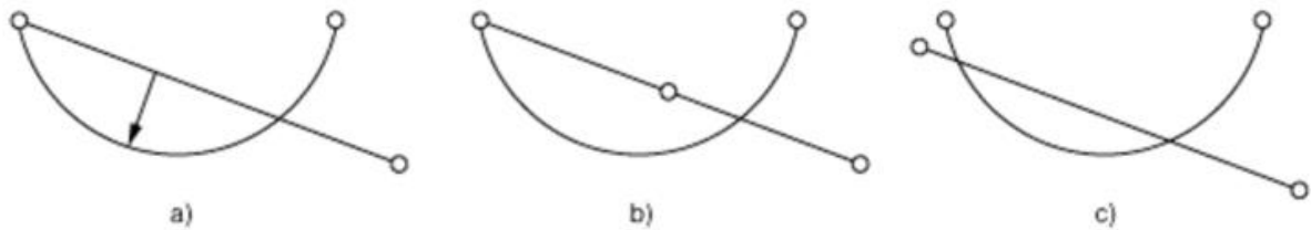
Figure 15: a) La flèche ne doit pas excéder la tolérance indiquée; b), c) recouvrements non permis pour une polygline, le segment de droite et l'arc de cercle en intersection n'ayant pas leur origine en un point d'appui commun.
