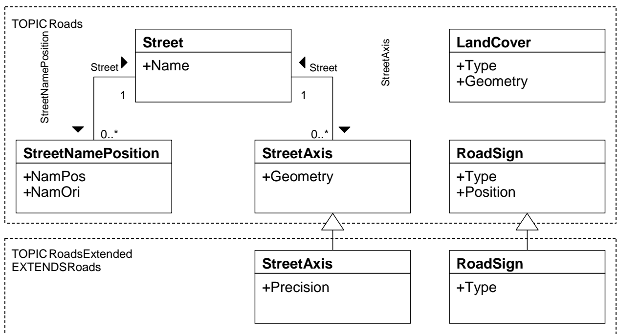
Figure 26: Diagramme de classe UML des modèles de données.
