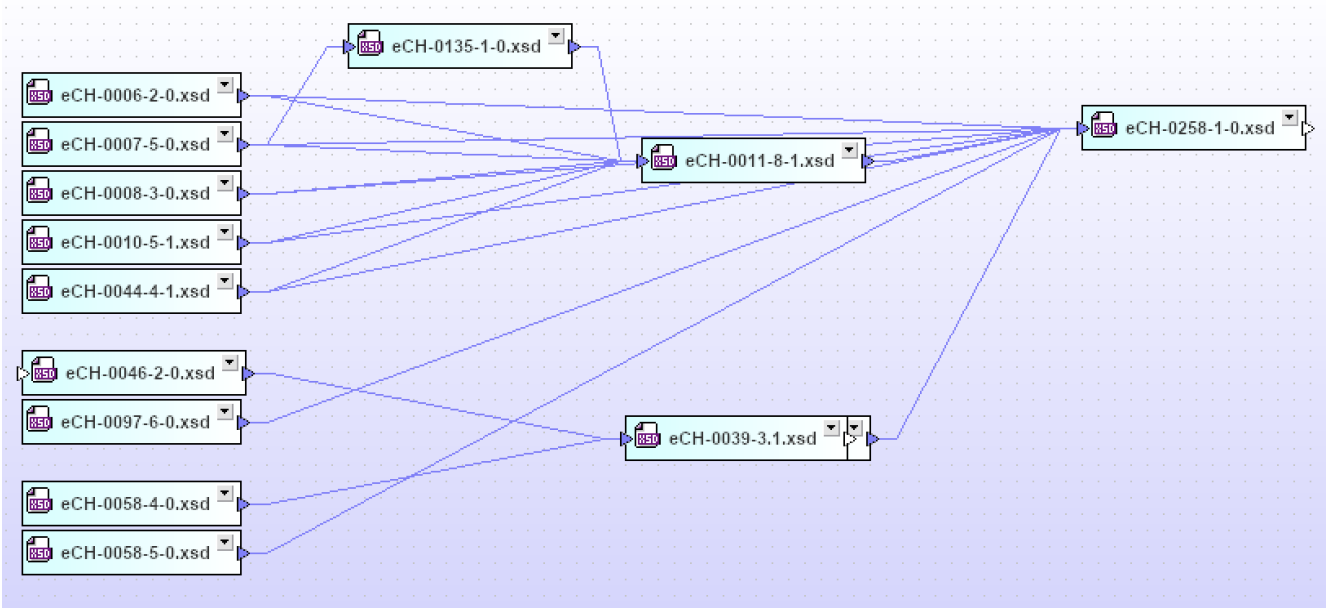
Figure 26: Dépendances
