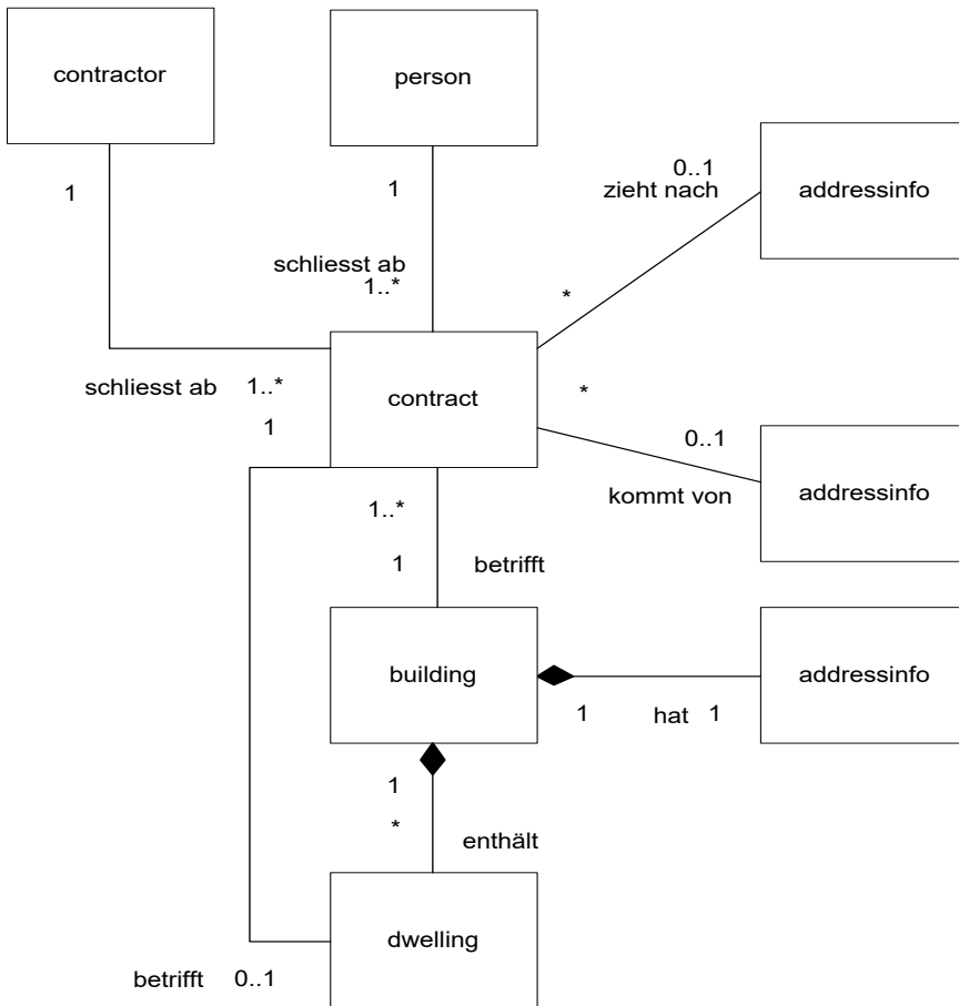
Abbildung 1: UML-Diagramm der übergebenen Fachdaten (vgl. [UML]).
