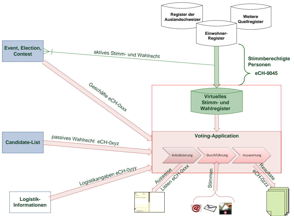
Figure 2: Disposition de l'eCH-0045
