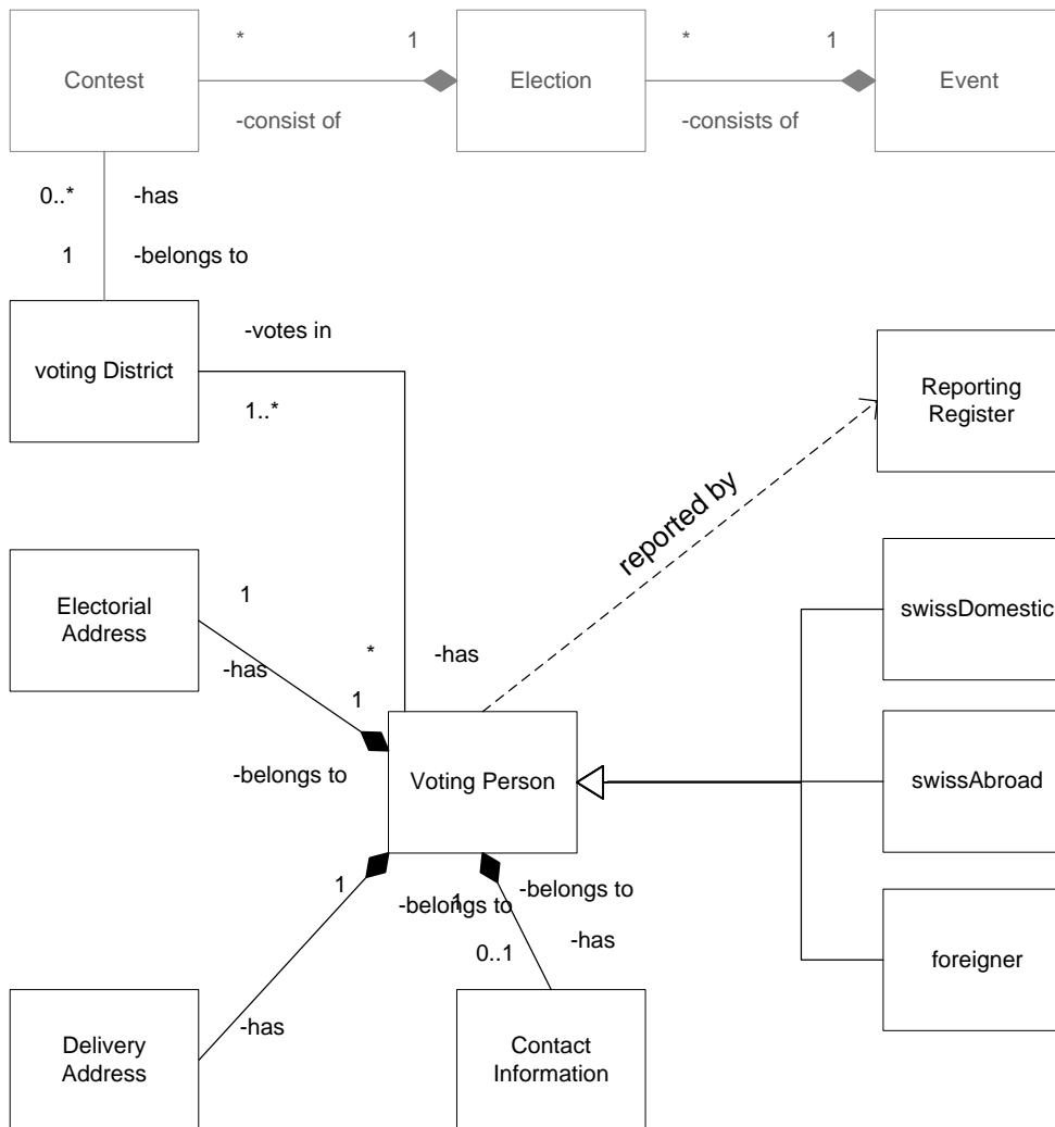
Figure 3: Modèle de données
