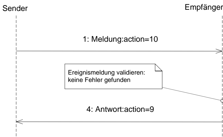
Abbildung 8: Weiterleitung
