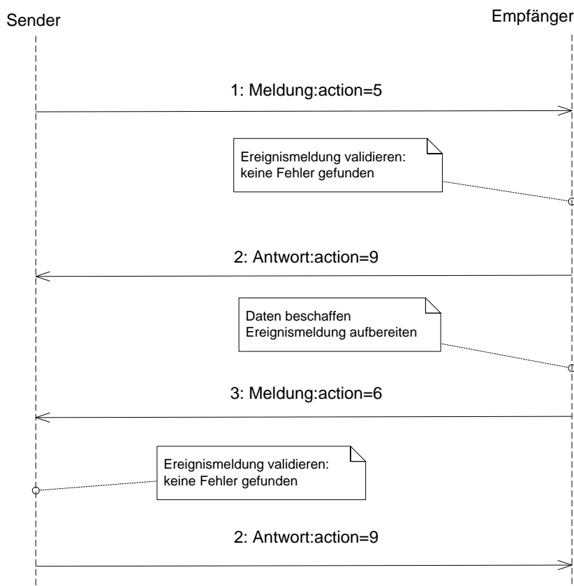
Abbildung 6: Datenanforderung
